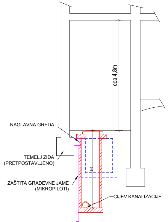
PRESJEK B
