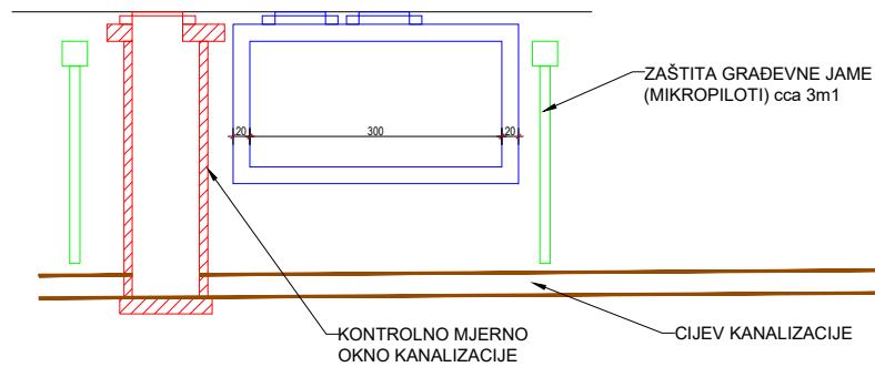
PRESJEK C
